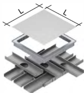
Dutos em níveis diferentes
