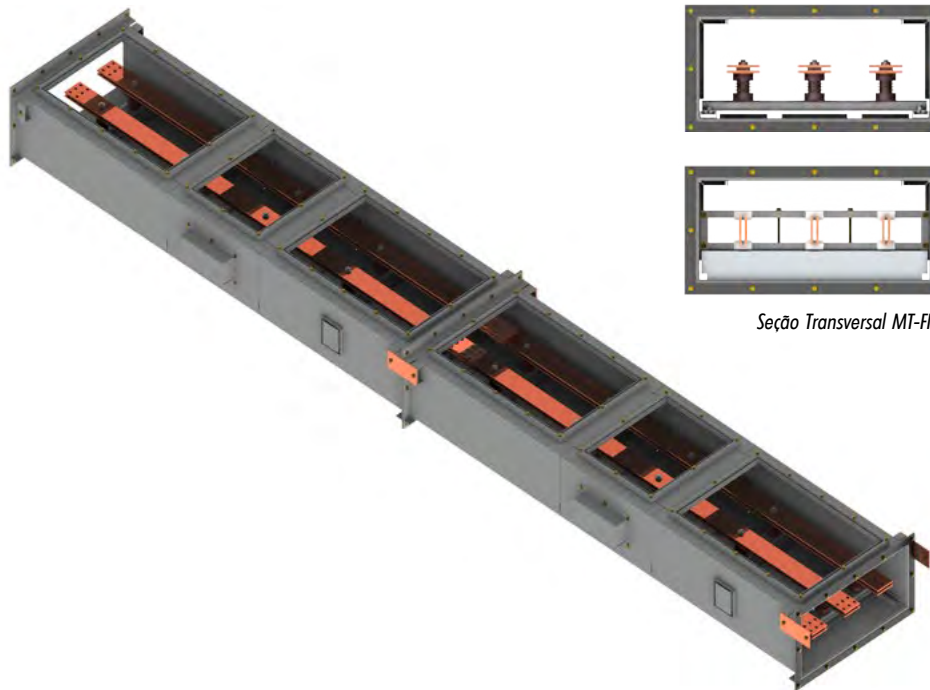
MT-FNS: Barramento de média tensão de fases não-segregadas
