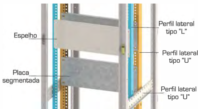
Placa de montagem segmentada e espelho interno fixados diretamente nos perfis verticais
