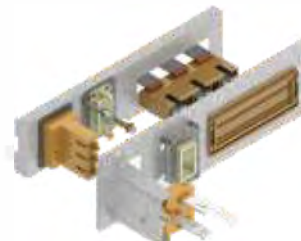
Entrada: Garra QT/Termofix Saída: Garra compacta Comando: Blocos Dock Frame
