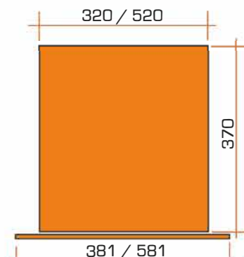
Dimensões da gaveta extraível interna
